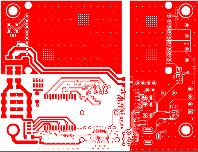
Top Layer (Scale 1:1)
