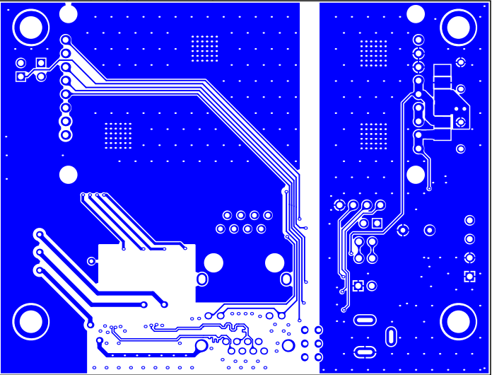
Bottom Layer (Scale 1:1)
