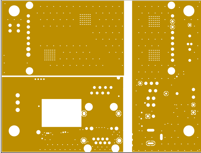
Layer 2 (Scale 1:1)
